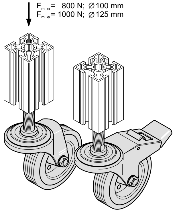
1 Lenkrolle mit Feststeller / Rollers with lock / Roulettes avec blocage / Rotella con bloccaggio / Ruedas con bloqueo
