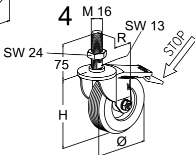
4 Rolle ohne Drehgelenk, mit Feststeller / Idle rollers, with lock / Roulettes non-dirigeable, avec blocage / Rotella senza snodo, con bloccaggio / Ruedas no-dirigibles, con bloqueo
